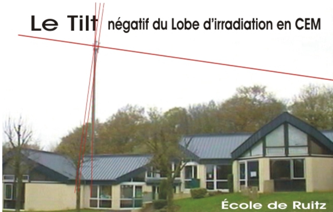
Les traits rouges matérialisent la direction des faisceaux des antennes situées sur le pylône.
